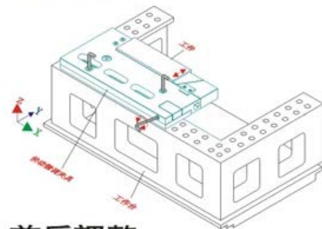
3. 前后調整
