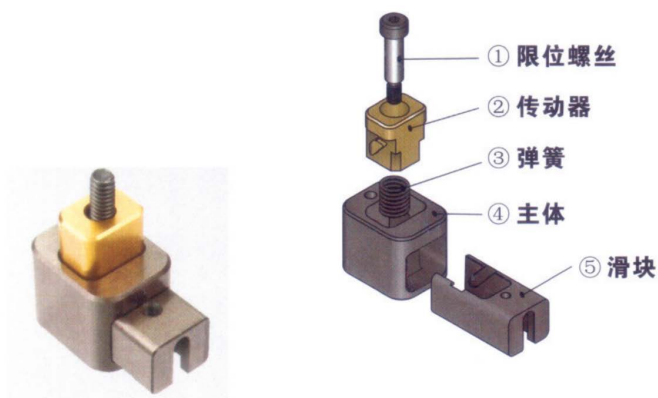
产品立体示意图:
