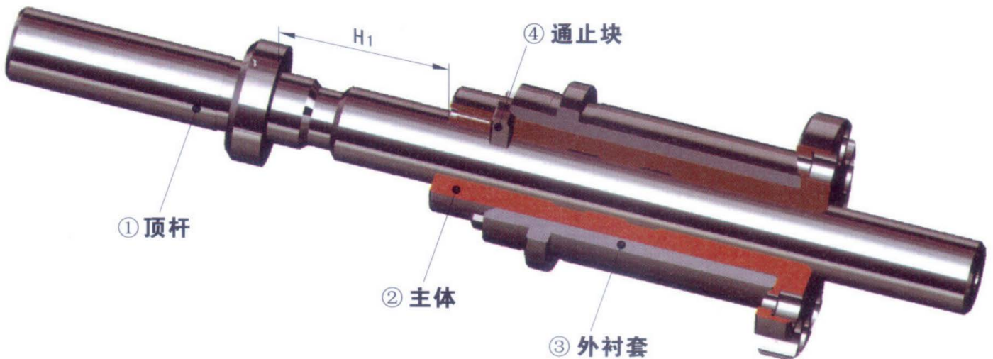
产品立体示意图:
